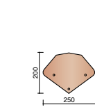
MK10 7070 Rive individuelle verticale droite (2,6 au ml)
