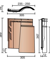
MK10 8112 Tuile 3/4 pureau (4,1 au ml)
